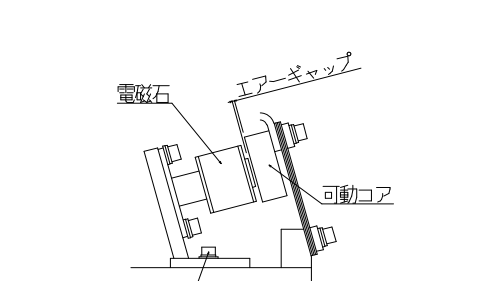
NV-3、4 エアーギャップ部詳細図
