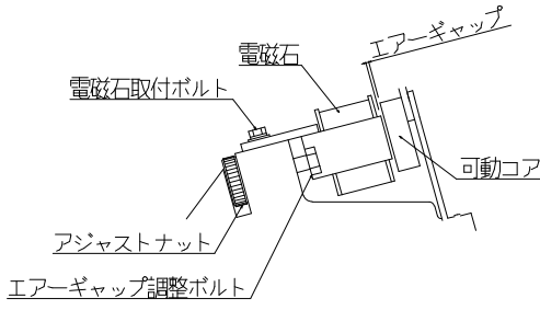
NV-2 エアーギャップ部詳細図
