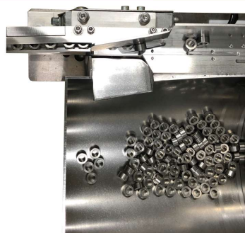
整列したワークを直進フィーダの振動で、出口まで送ります。 それ以外のワークはドラム内に戻ります。
